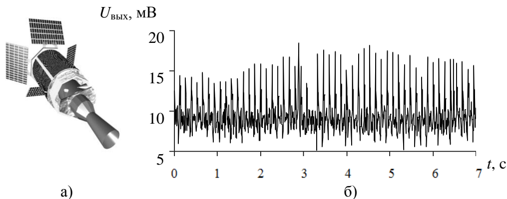
Рис. 5. Типовой ГСС [2]: а – предполагаемый внешний вид типового ГСС; б – фотометрическая кривая блеска типового ГСС
