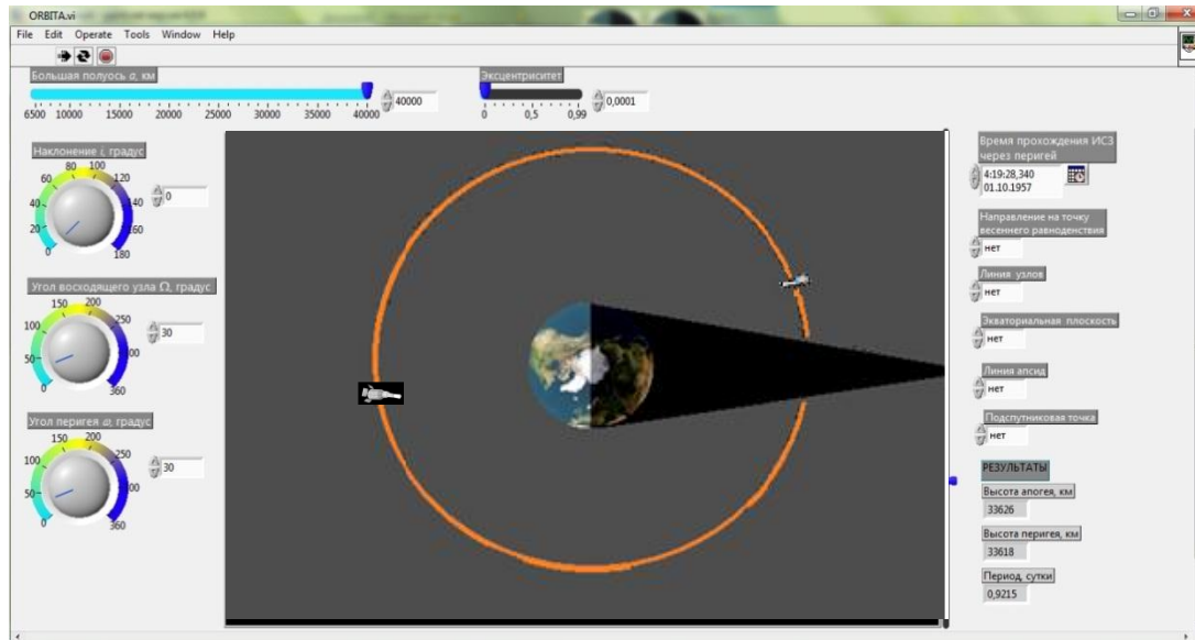
Рис. 3. Условия оптической видимости ИСЗ (масштаб не соблюден)
