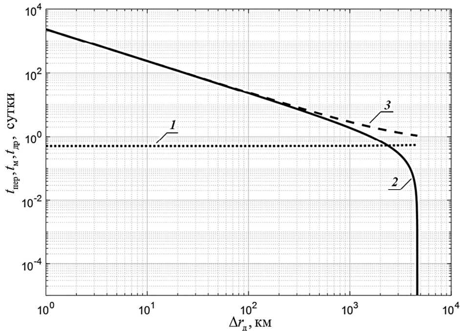
Рис. 3. Зависимость времен перелета, маневра и дрейфа для различных орбит дрейфа: 1 – время маневра t_{\text{м}} ; 2 – время дрейфа t_{\text{др}} ; 3 – время перелета t_{\text{пер}}
