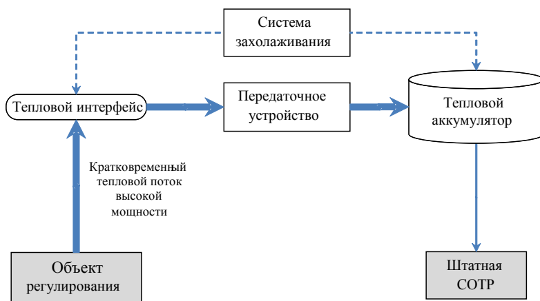
Рис. 1. Принципиальная схема специальной СОТР
